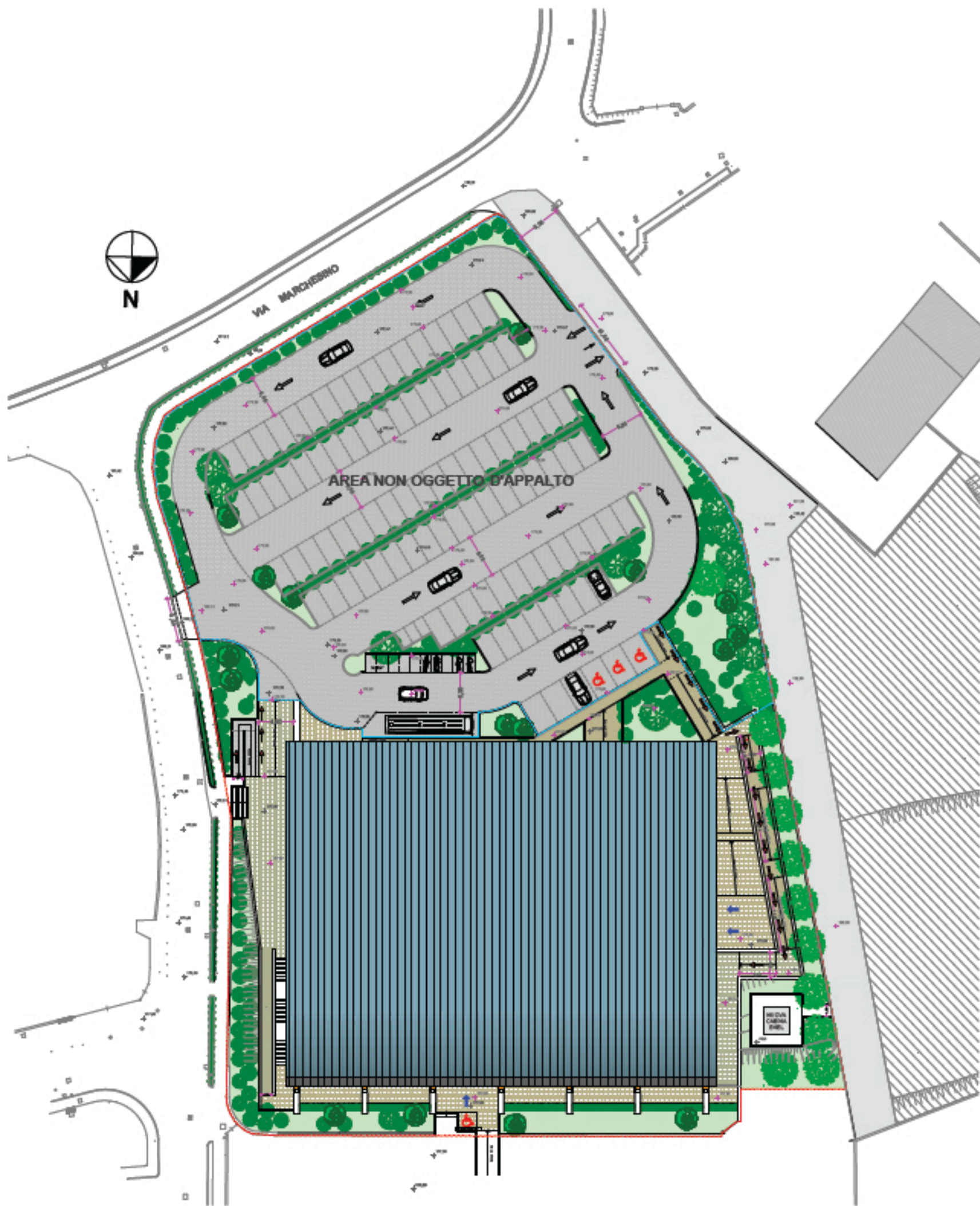
PLANIMETRIA GENERALE Scala 1:200
